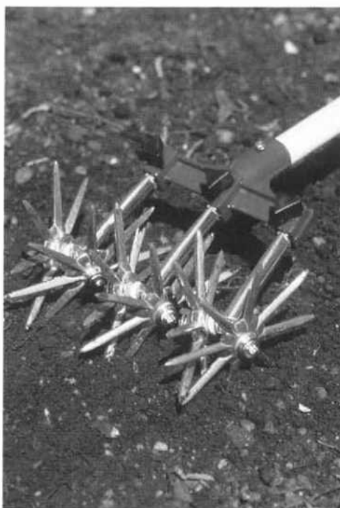
Mit den rotierenden Werkzeugen der Sternfräse wird der Boden gelüftet, gelockert und z. T. auch von Unkraut befreit.
