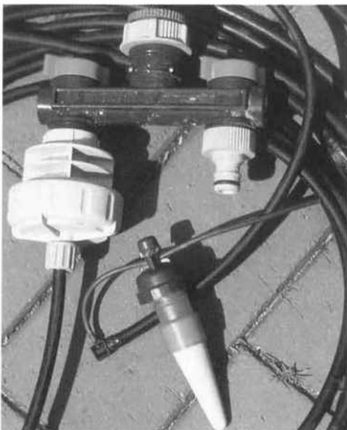
Ausrüstung einer automatischen Bewässerung: 2-Wege-Verteiler, Druckminderer, Hauptschlauch, Tonkegel und Tropfschlauch.
